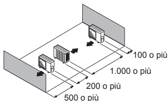
(1) Disposizione unità in parallelo singola
