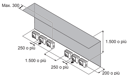
(1) Disposizione unità in parallelo singola
