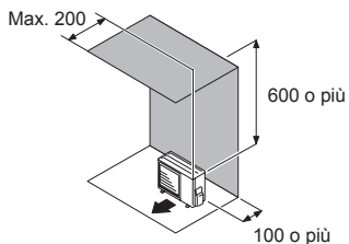
(1) Ostacoli nella parte posteriore e superiore
