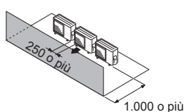
(2) Ostacoli sono nella parte anteriore
