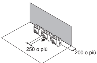
(3) Ostacoli nella parte anteriore e posteriore
