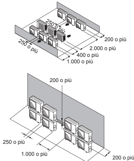
(2) Disposizione unità in parallelo multipla
