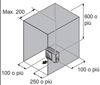
(2) Ostacoli nella parte posteriore, laterale e sopra
