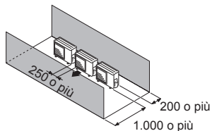
(3) Ostacoli nella parte anteriore e posteriore
